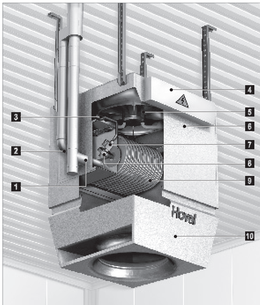
Fig. C1: TopVent® DGV estructura
