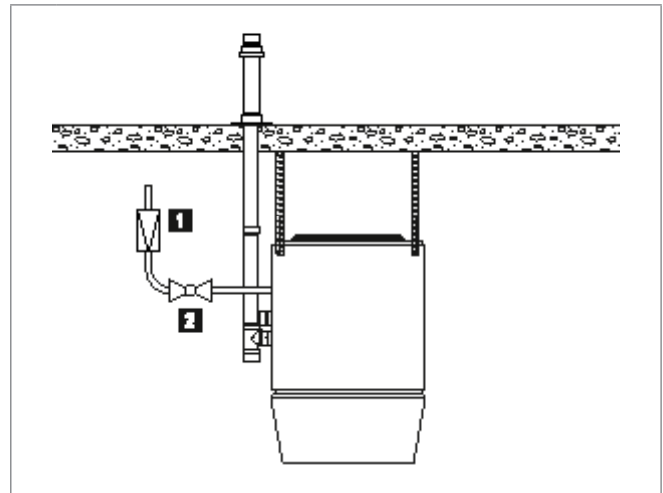
1 Regulador presión del gas (20...50 mbar)
